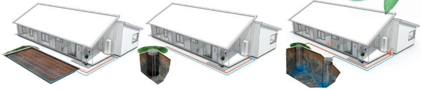
Wärmepumpe mit Flachkollektor
